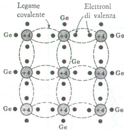
Fig. 3. - Rappresentazione simbolica in due dimensioni della struttura cristallina del Ge.
