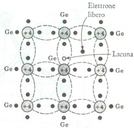
Fig. 4. - Cristallo di Ge con un legame covalente rotto.
